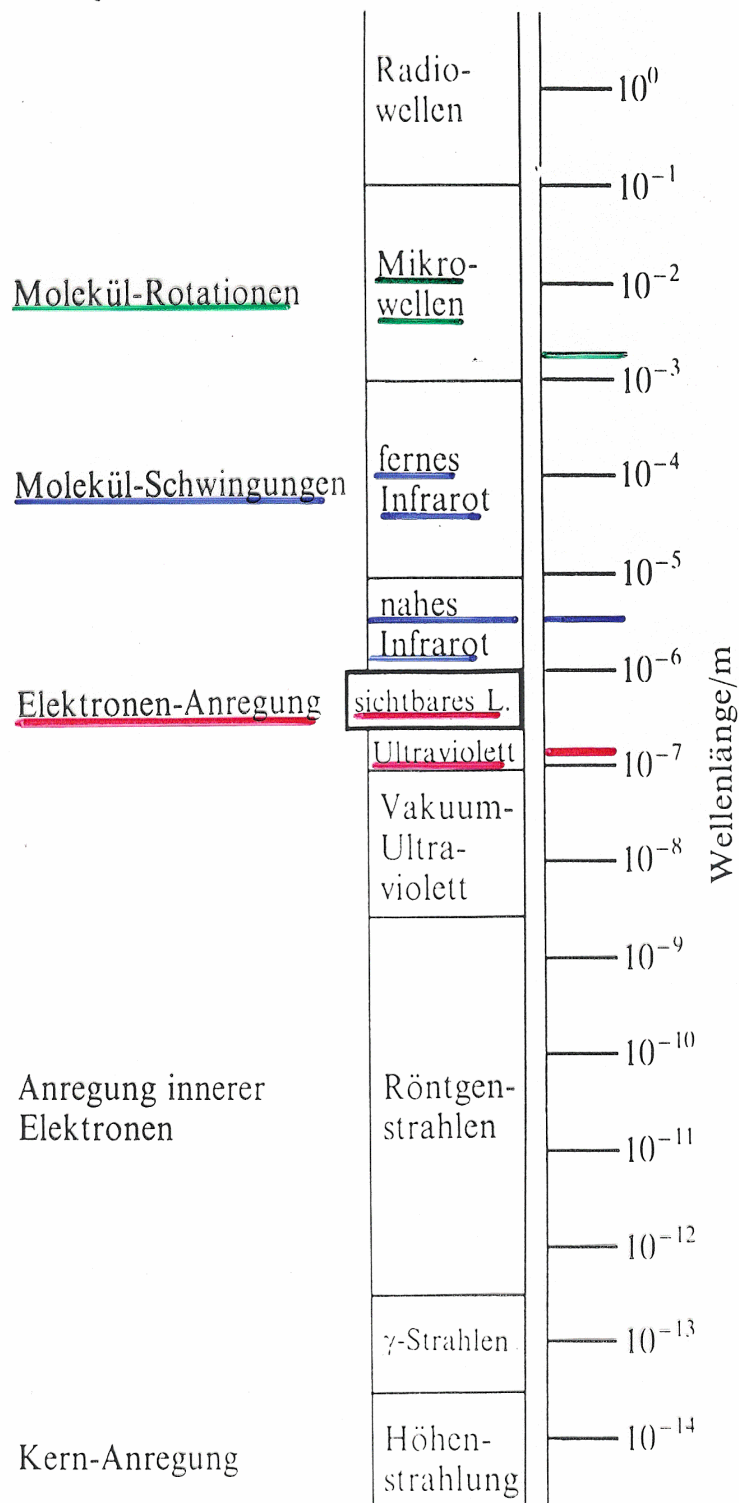
Abb. 0-6 Die Einteilung der verschiedenen Bereiche des elektromagnetischen Spektrums nach der Wellenlänge der Strahlung. Beachten Sie, daß zu den kürzeren Wellenlängen die energiereicheren Quanten gehören.
